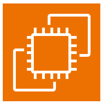
EC2
