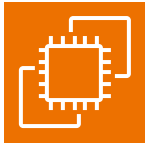
EC2
