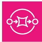
SQS
