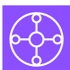
TransitGateway
